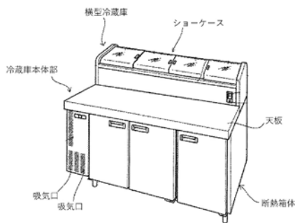
【概略斜視図】
